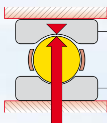
Рабочий радиальный зазор
