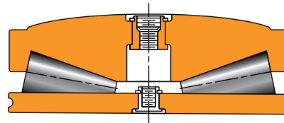
Fig. 12. Type TTHDFLSX.
