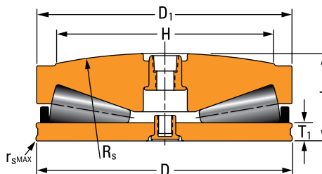
Fig. 91. Type TTHDFLSX-2.
