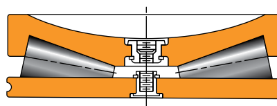
Fig. 13. Type TTHDFLSV.
