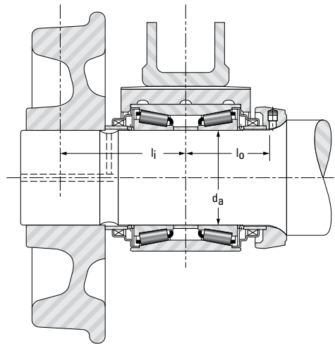
Inboard Journal
