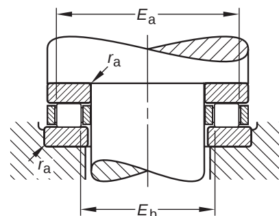
Way contact dimensions
