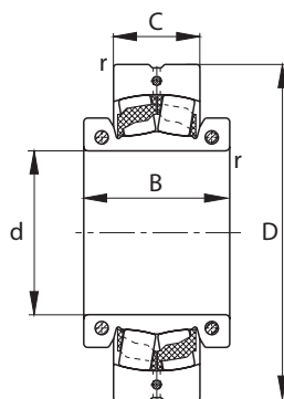
Массивный сепаратор из полиамида TVPA
