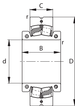
Массивный сепаратор из полиамида TVPA
