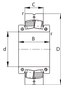
Массивный сепаратор из латуни МА
