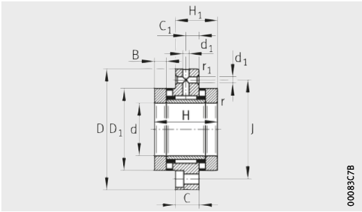
ZARF
