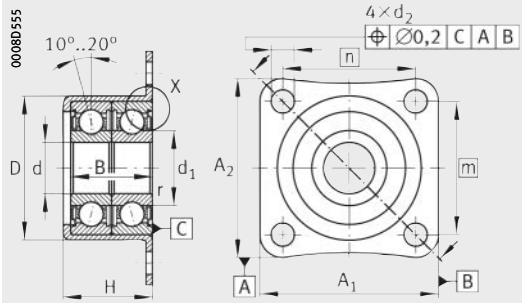
ZKL1035-2Z
