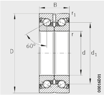
ZKLN...-2RS-PE
