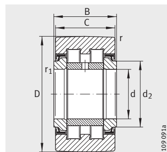
PWTR..-2RS (с оптимизированным профилем INA)
