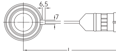
BMB ... 108A (Supersea™) BMO ... 008A (Supersea™)
