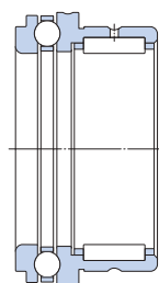
NKX ( F_w \geq 12 mm)
