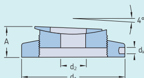
Низкопрофильное исполнение SKF Vibracon
