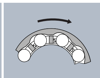
Figure 2 Roue libre tournant à vide
