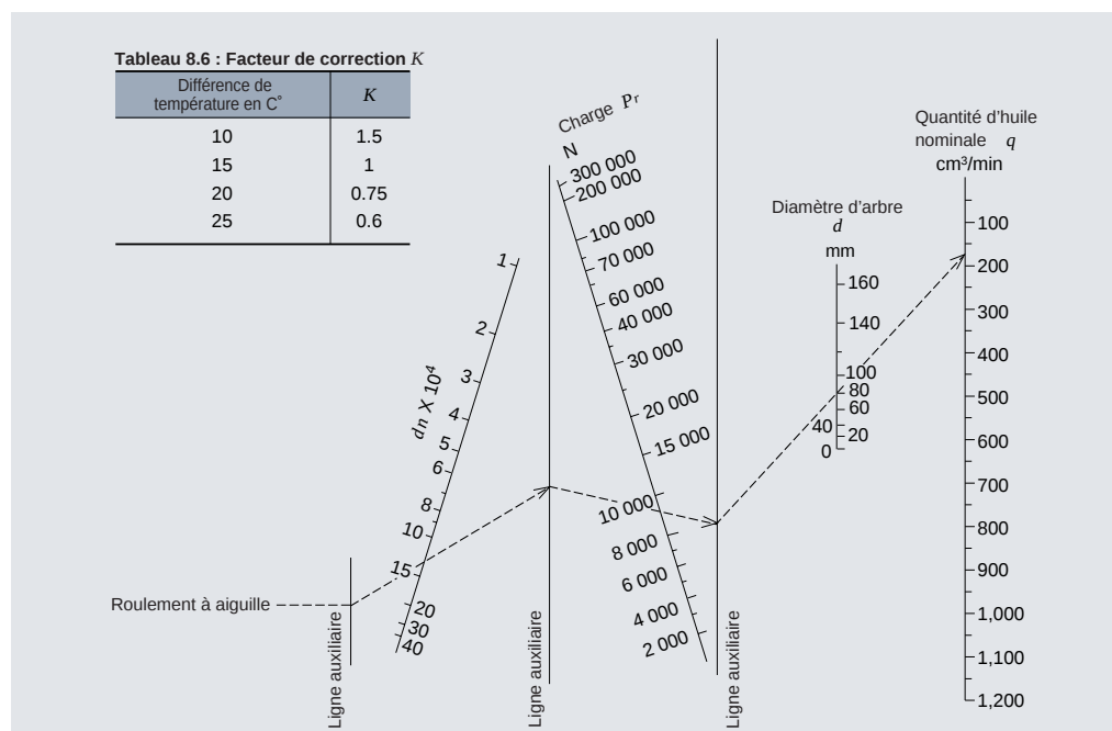
Figure 8.6 : Diagramme pour détermination de la quantité d'huile
