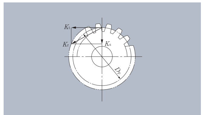
Figure 3.3 : Résultante sur engrenage
