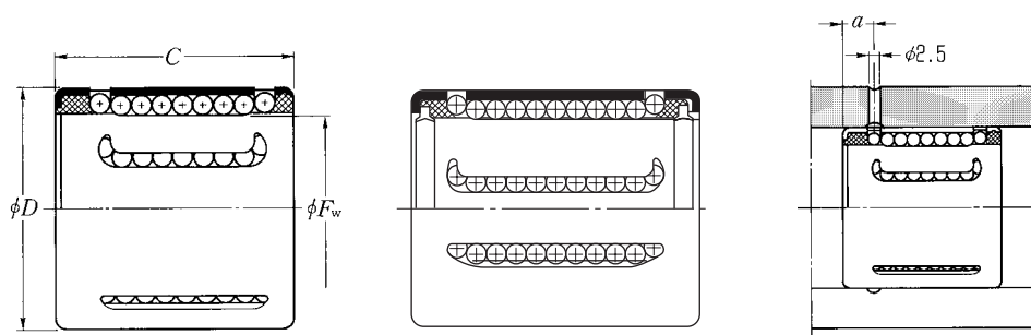
Avec étanchéité
