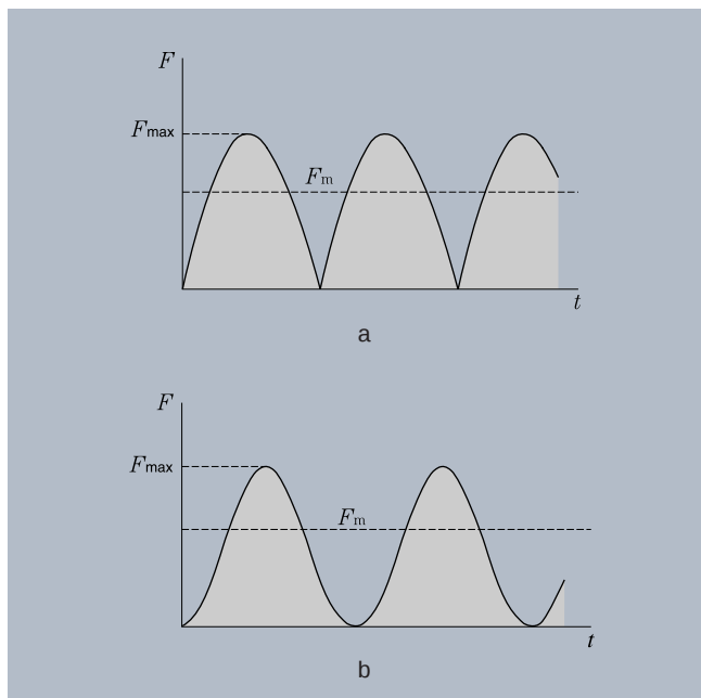
Figure 3.11 : Variation sinusoïdale de la charge
