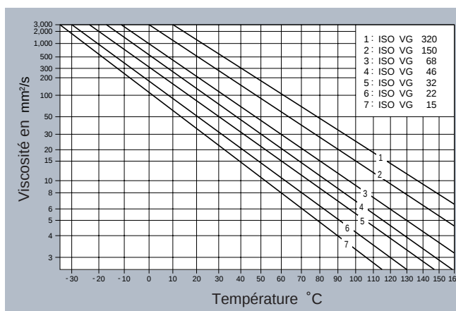
Figure 8.5 : Diagramme viscosité-température
