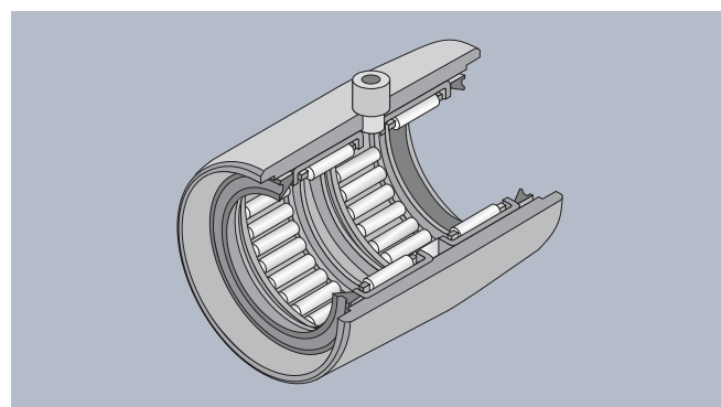
Figure 4 : Série FR
