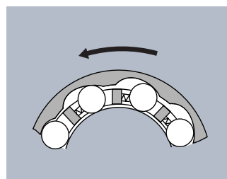
Figure 1 Roue libre enclenchée
