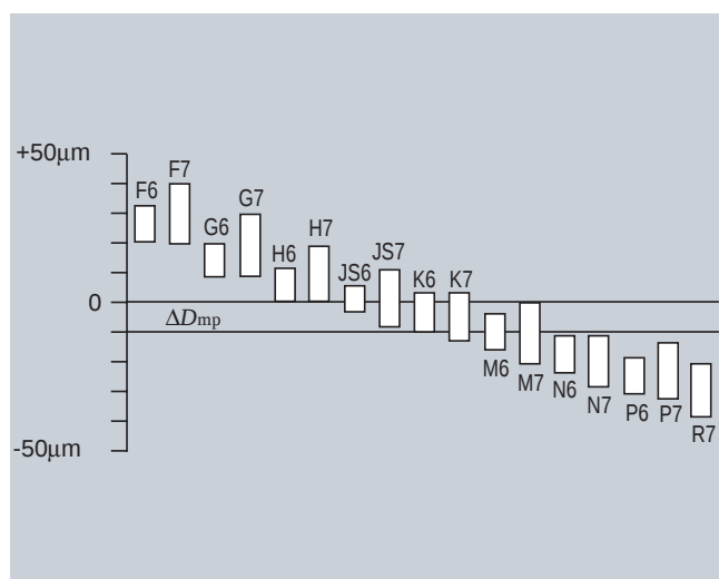
Figure 6.1 (b) : Ajustements dans le logement
