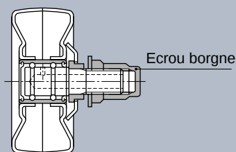
Fig. 3 Galet tendeur à double rangée de billes
