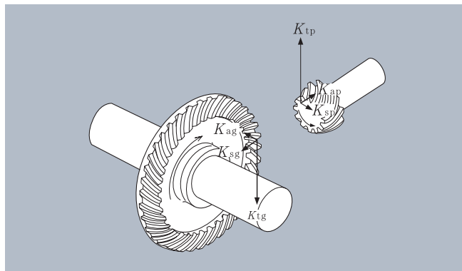
Figure 3.4 : Efforts sur roues dentées coniques
