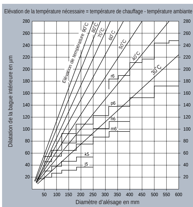
Figure 10.3 : Elévation de température nécessaire pour montage à chaud
