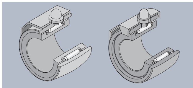
Figure 1 : Série FRIS · SA
