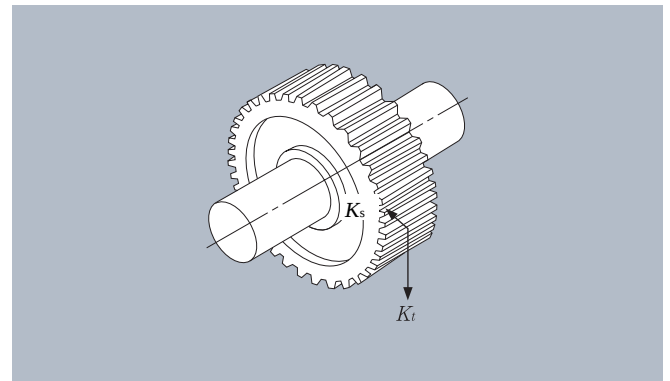
Figure 3.1 : Efforts sur roues dentées droites
