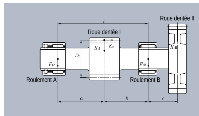
Figure 3.7 : Arbre de transmission
