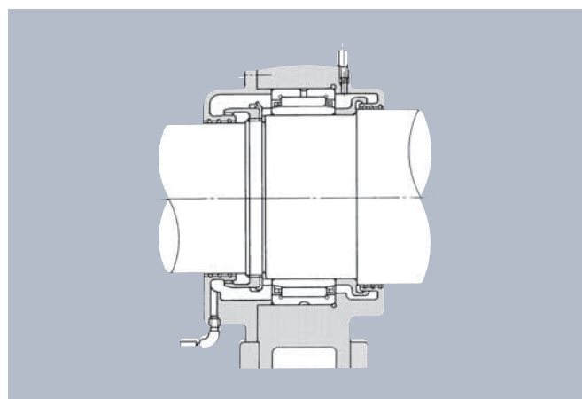
Figure 8.4 : Lubrification par circulation d'huile
