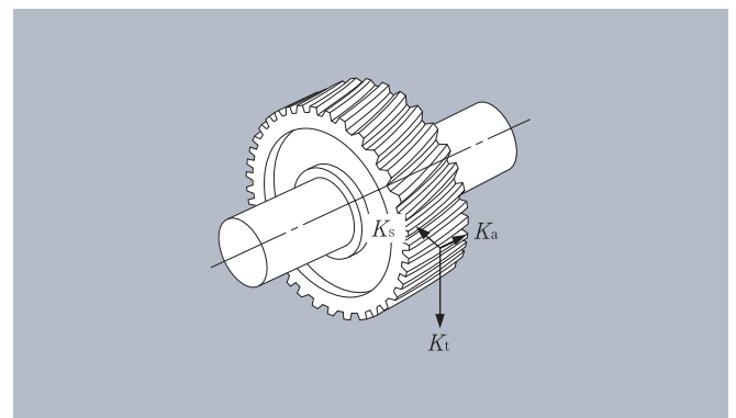
Figure 3.2 : Efforts sur roues dentées hélicoïdales
