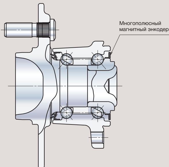
Рис. 11. Пример устройства осевого типа
