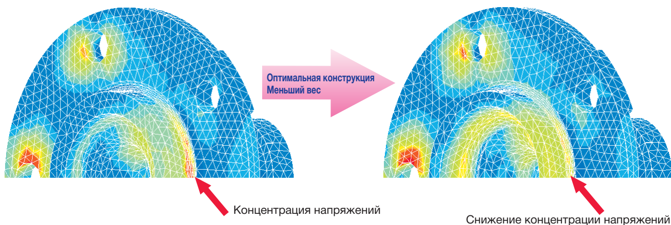
Рис.5. Пример АМКЭ (Внутренний фланец)
