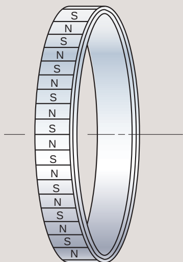
Рис. 10. Пример устройства радиального типа
