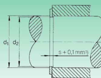
Einbaumaße Монтажные размеры
