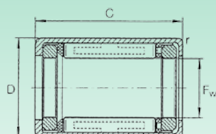
HFL, HFL..KF mit Gleitlager HFL, HFL..KF со скользящим подшипником
