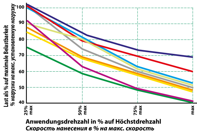
Belastbarkeit/Geschwindigkeit Мощность/Скорость
