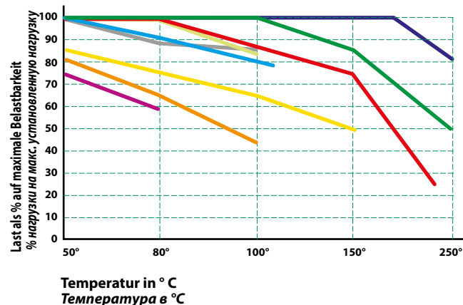
Belastbarkeit/Temperatur Мощность/Температура
