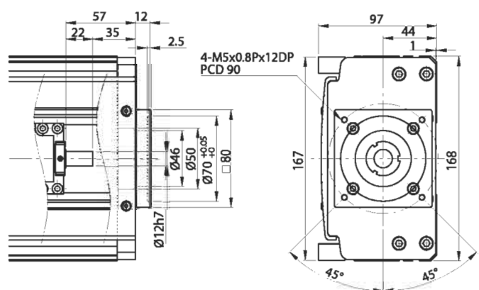
Переходный фланец двигателя F2
