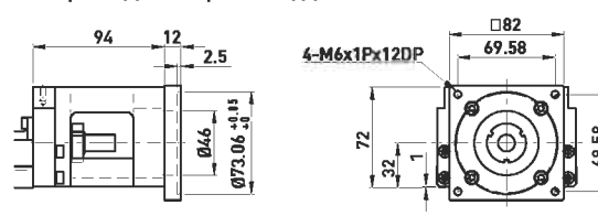
Переходный фланец двигателя F4
