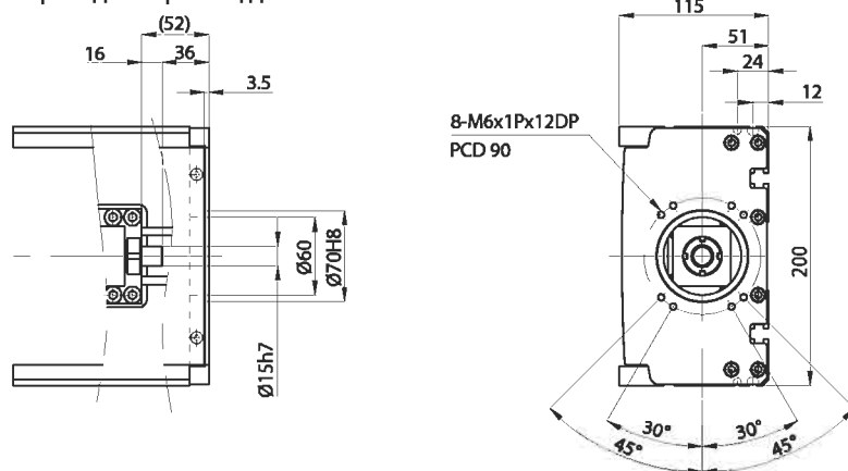
Переходный фланец двигателя F1
