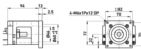
Переходный фланец двигателя F4
