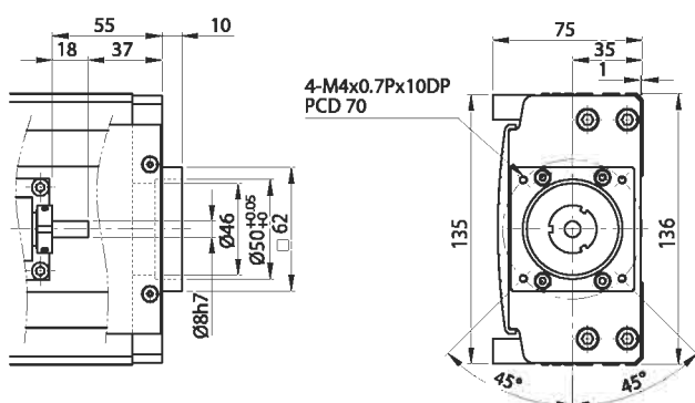
Переходный фланец двигателя F2
