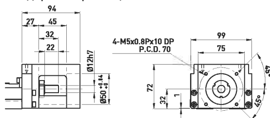
Переходный фланец двигателя F1
