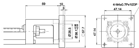
Переходный фланец двигателя F5
