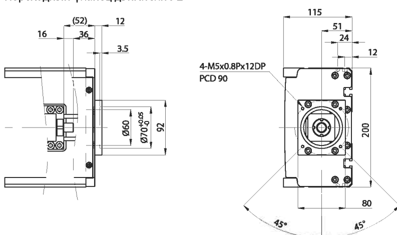
Переходный фланец двигателя F2
