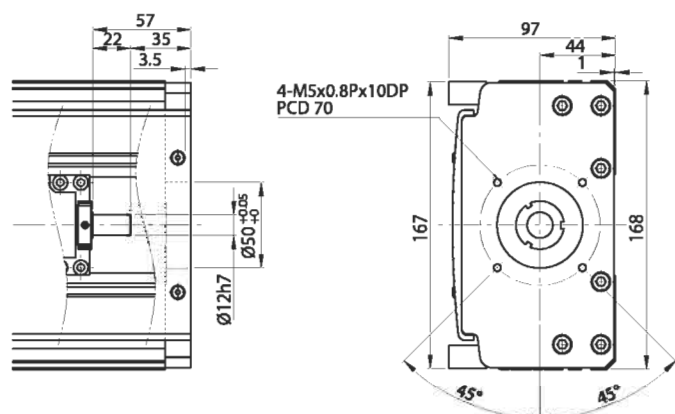
Переходный фланец двигателя F0
