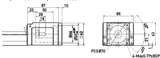
Переходный фланец двигателя F2
