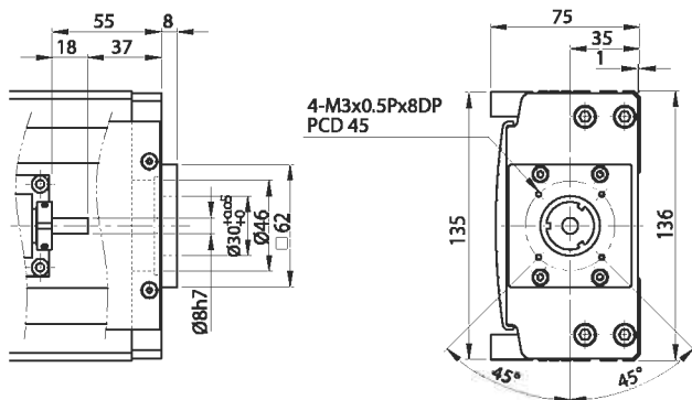
Переходный фланец двигателя F3
