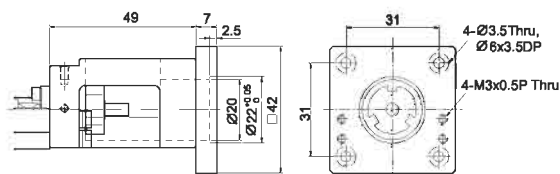
Переходный фланец двигателя F3
