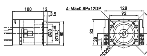
Переходный фланец двигателя F4
