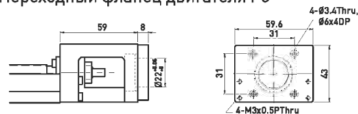
Переходный фланец двигателя F5
