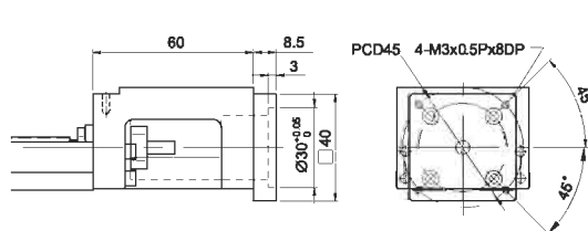
Переходный фланец двигателя F3
