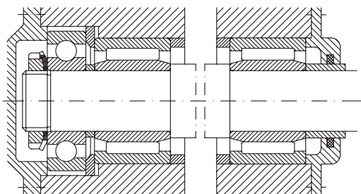
фиксированного подшипника f) свободного подшипника
